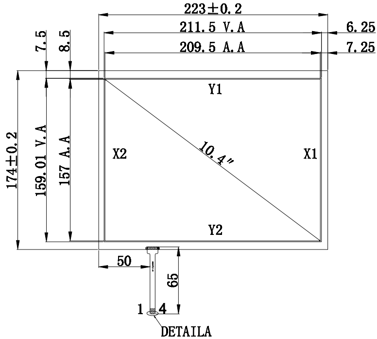
正视图
