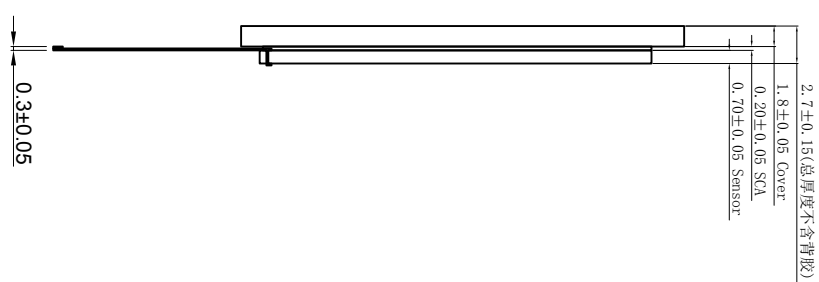
侧视图 横向10:1
